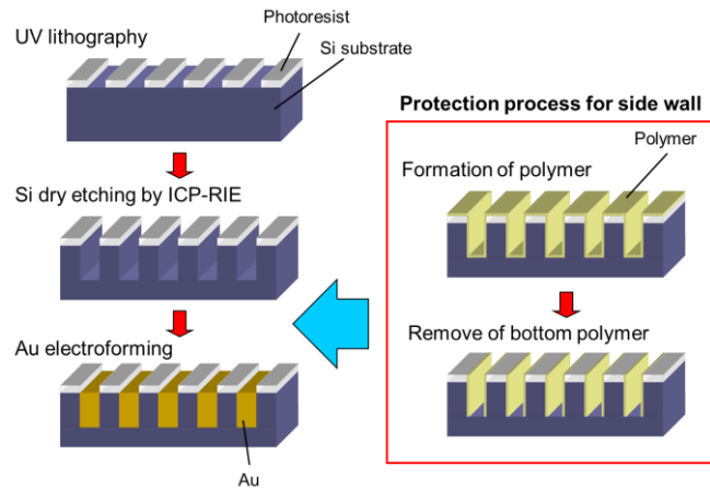
Fig. 3: Fabrication process of Au microstructures.
