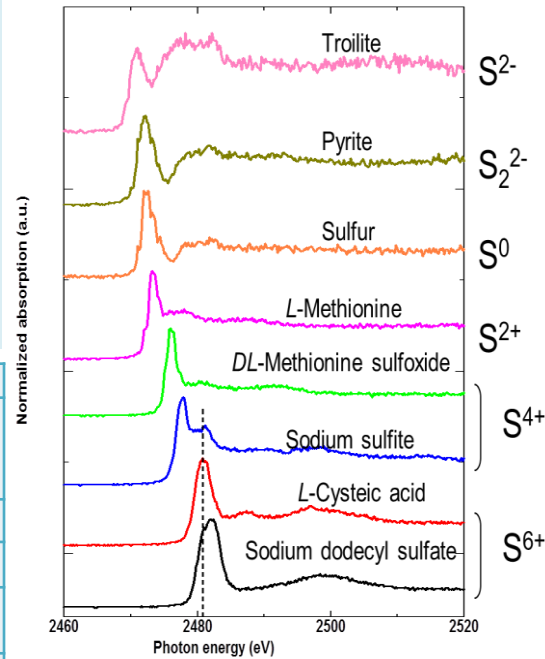
XAFSスペクトル S-K端
